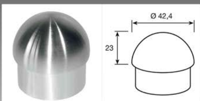
EX155 TAPPO BOMBATO Ø 42,4 - INOX AISI 304 SATINATO
