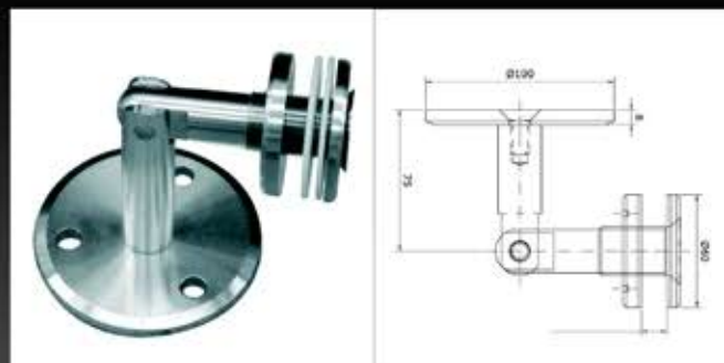
EX740 ATTACCO INFERIORE AISI 304 PER PENSILINA
