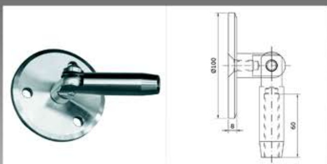
EX745 ATTACCO SUPERIORE AISI 304 PER PENSILINA
