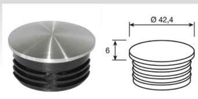
EX140 KIT TAPPO PIANO DN 42,4 PLASTICA E ACCIAIO SATINATO
