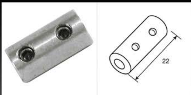
EX420 FERMO 4 mm - INOX AISI 304
