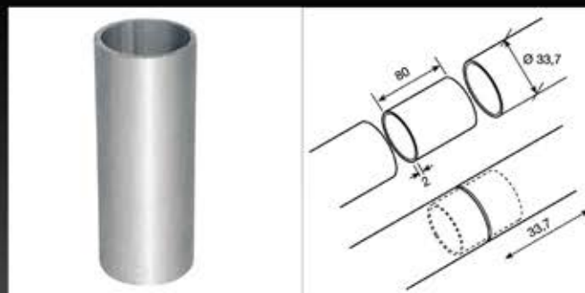
EX290 INNESTO DI GIUNZIONE \varnothing 33,7 - INOX AISI 304
