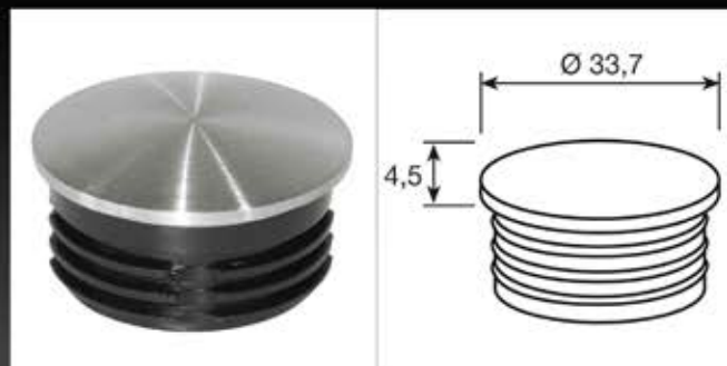
EX120 KIT TAPPO PIANO DN 33,7 PLASTICA E ACCIAIO SATINATO
