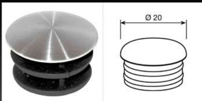
EX115 KIT TAPPO PIANO DN 20 PLASTICA E ACCIAIO SATINATO
