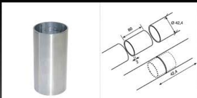
EX280 INNESTO DI GIUNZIONE \varnothing 42,4 - INOX AISI 304
