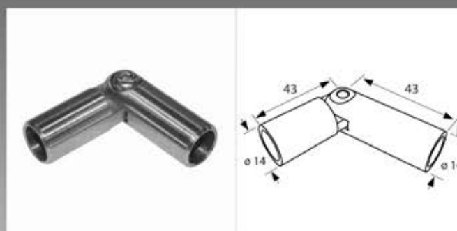
EX252 SNODO 12 - INOX AISI 304 SATINATO
